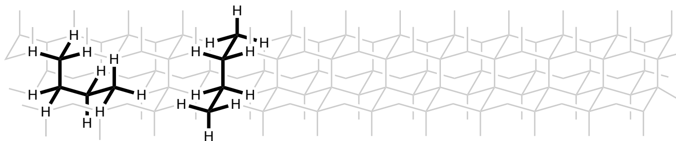
gauche butane
