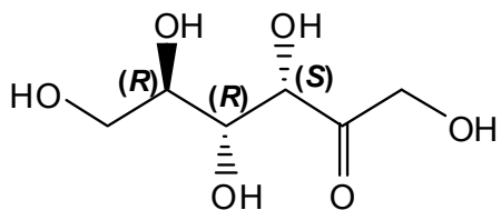
D-fructose
